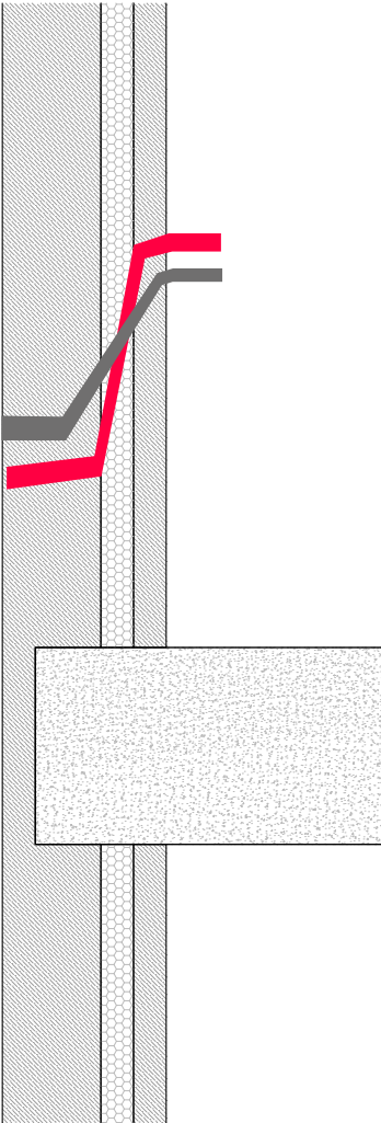
FACHADA CON DOBLE MURO DOUBLE-BRICK FACADE
