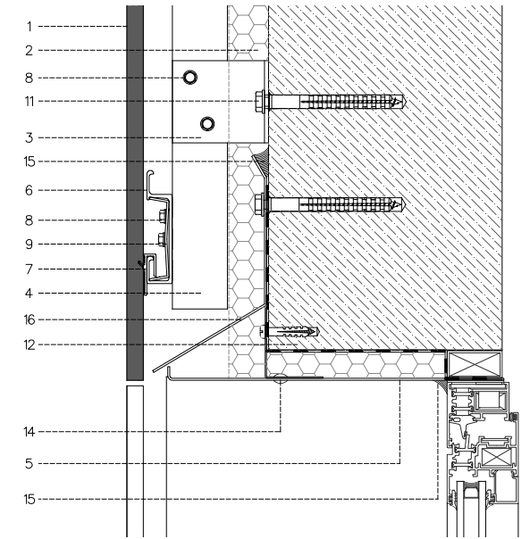
DINTEL METÁLICO METAL LINTEL
