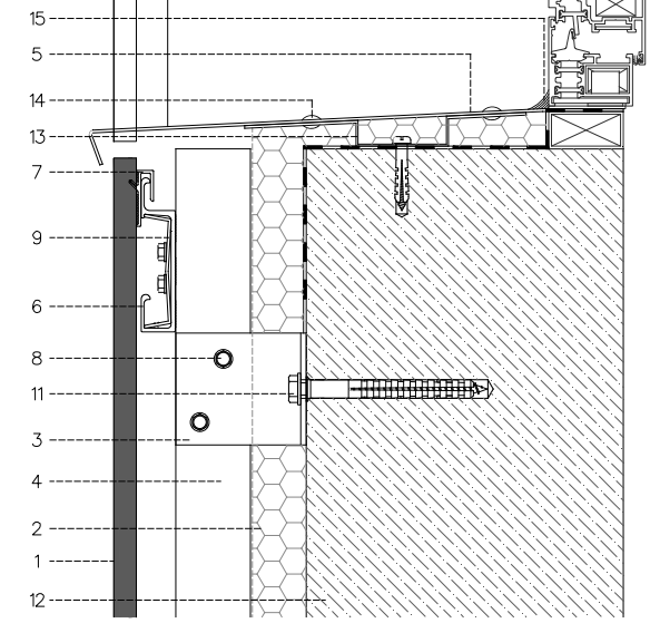
VIERTEAGUAS METÁLICO METAL FLASHING
