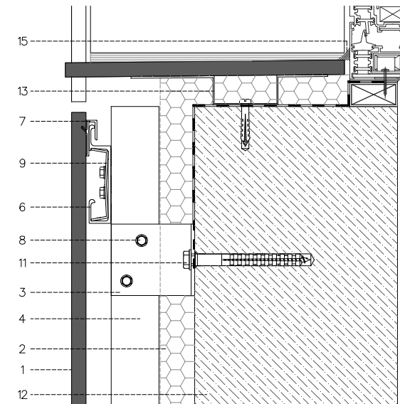
VIERTEAGUAS CERÁMICO CERAMIC FLASHING
